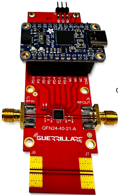
GRF6403
